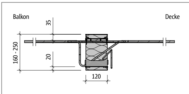
Abb. 84: Schöck Isokorb® XT Typ K-ID-M3 bei R0: Produktschnitt
