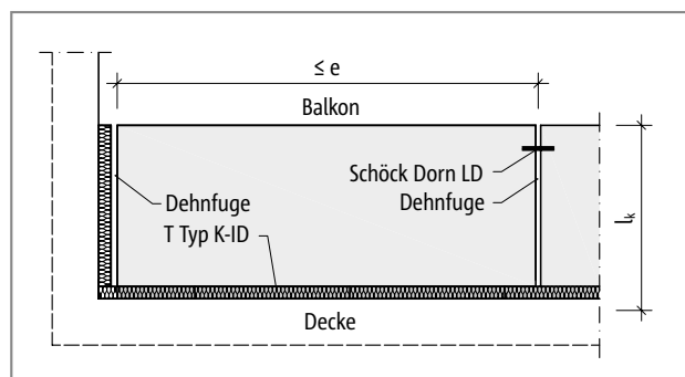
Abb. 110: Schöck Isokorb® T Typ K-ID: Dehnfugenanordnung
