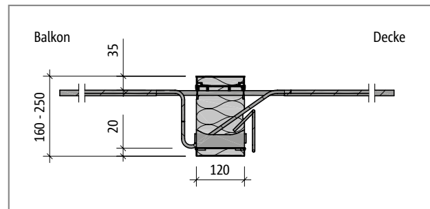
Abb. 85: Schöck Isokorb® XT Typ K-ID-M4 bei R0: Produktschnitt
