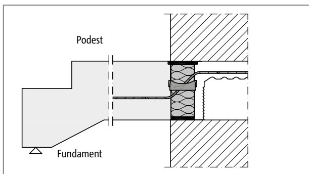
Abb. 169: Schöck Isokorb® T Typ Q-ID: Anschluss Treppenlauf bei monolithischem Mauerwerk
