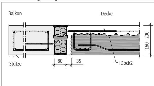
Abb. 171: Schöck Isokorb® T Typ Q-ID: Anschluss von Balkonen mit Plattendicken von 160 mm bis 200 mm mit IDock2
