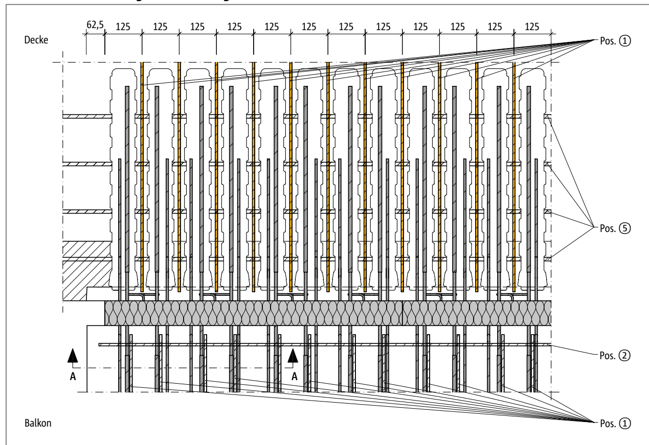
Abb. 129: Schöck Isokorb® T Typ K-ID: Achsmaß der bauseitigen Bewehrung im Grundriss
