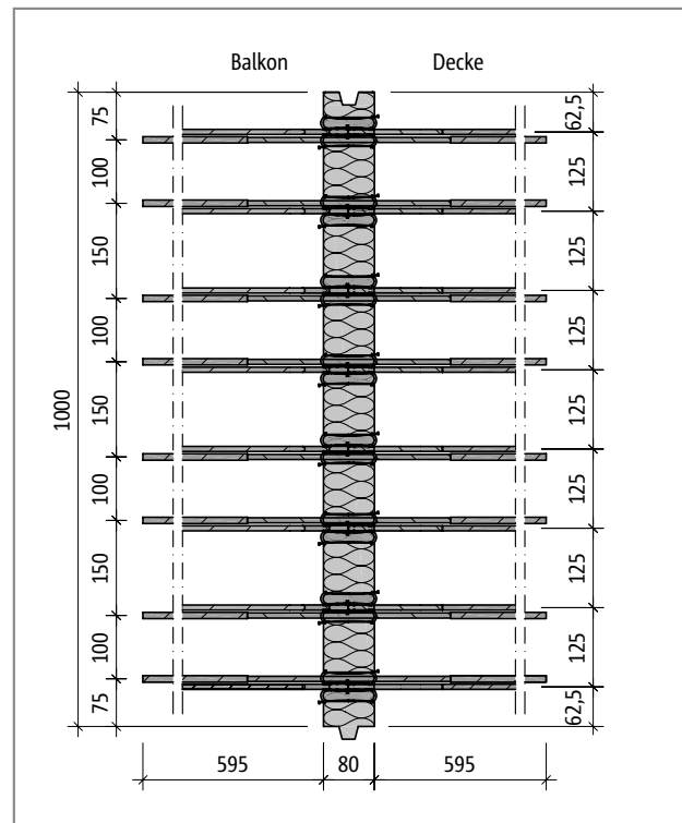
Abb. 120: Schöck Isokorb® T Typ K-ID-M2-V2-R0-X80: Produktgrundriss
