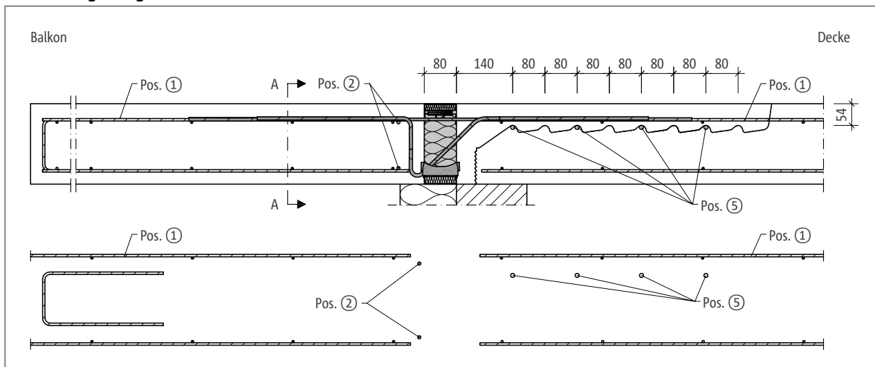
Abb. 131: Schöck Isokorb® T Typ K-ID: Bauseitige Bewehrung bei direkter Lagerung
