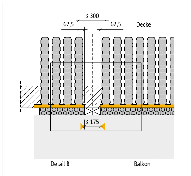
Abb. 178: Schöck Isokorb® T Typ Q-ID: Anordnung einer Aussparung in der Dämmebene mit einer gewählten Länge \leq 175 mm
