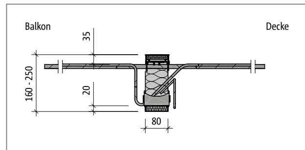
Abb. 122: Schöck Isokorb® T Typ K-ID-M4: Produktschnitt
