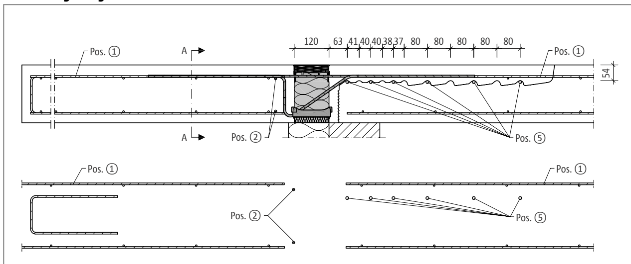
Abb. 89: Schöck Isokorb® XT Typ K-ID: Bauseitige Bewehrung bei direkter Lagerung
