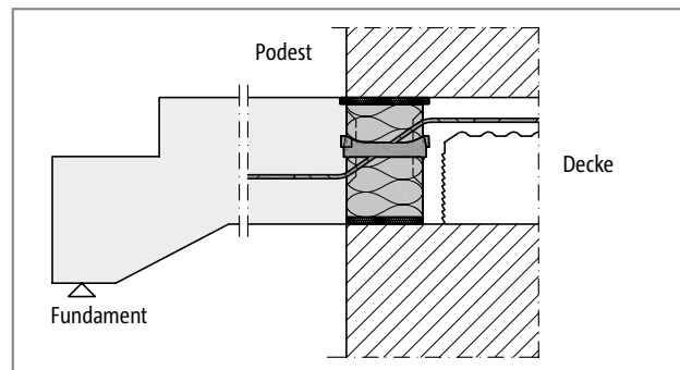
Abb. 141: Schöck Isokorb® XT Typ Q-ID: Anschluss Treppenlauf bei monolithischem Mauerwerk
