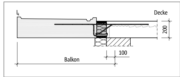
Abb. 94: Schöck Isokorb® XT Typ K-ID: Statisches System
