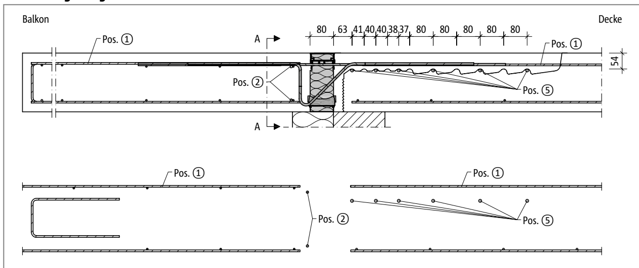
Abb. 132: Schöck Isokorb® T Typ K-ID: Bauseitige Bewehrung bei direkter Lagerung
