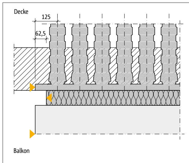
Abb. 111: Schöck Isokorb® T Typ K-ID: Randabstand des Dämmkörpers, Achsmaß der Deckenaussparungen; Darstellung im Grundriss
