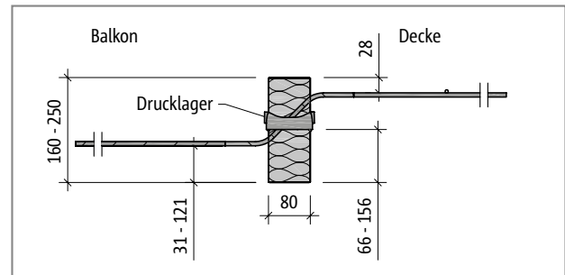
Abb. 185: Schöck Isokorb® T Typ Q-ID-V4-R0-X80: Produktschnitt
