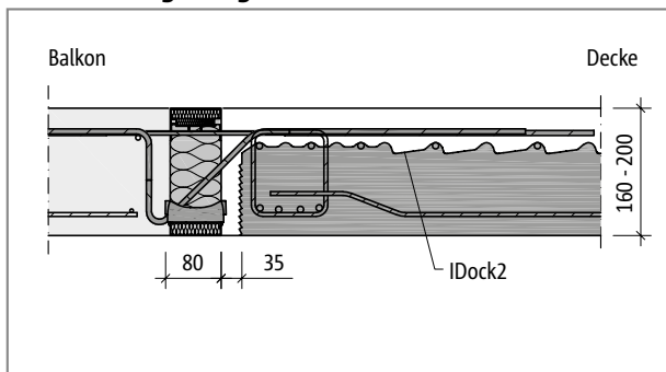
Abb. 106: Schöck Isokorb® T Typ K-ID: Anschluss von Balkonen mit Plattendicken von 160 mm bis 200 mm mit IDock2
