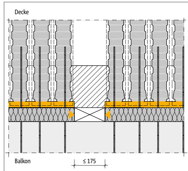
Abb. 179: Schöck Isokorb® T Typ Q-ID: Detail B, richtig durch Einhaltung der vorgegebenen Abstände und der Aussparungslänge \leq 175 mm
