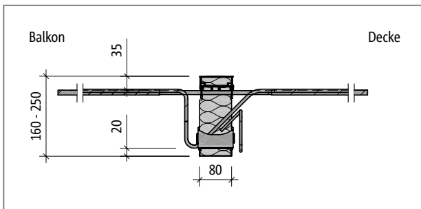
Abb. 127: Schöck Isokorb® T Typ K-ID-M3-V2-R0-X80: Produktschnitt
