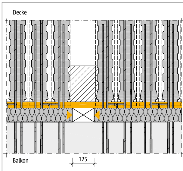
Abb. 114: Schöck Isokorb® T Typ K-ID: Detail A, richtig durch Einhaltung des Rastermaßes und der vorgegebenen Abstände
