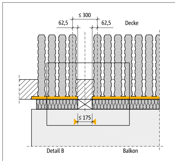
Abb. 150: Schöck Isokorb® XT Typ Q-ID: Anordnung einer Aussparung in der Dämmebene mit einer gewählten Länge \leq 175 mm
