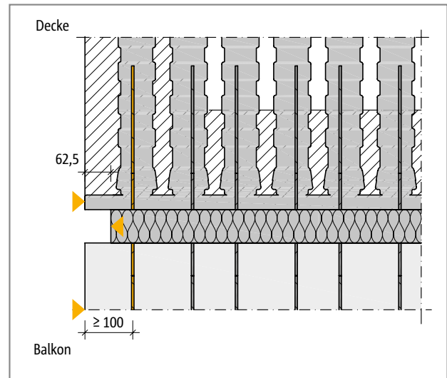
Abb. 175: Schöck Isokorb® T Typ Q-ID: Randabstand des Dämmkörpers, Mindestrandabstand des Querkraftstabs; Darstellung im Grundriss
