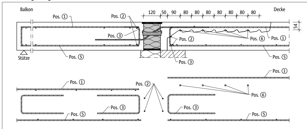
Abb. 159: Schöck Isokorb® XT Typ Q-ID: Bauseitige Bewehrung bei direkter Lagerung
