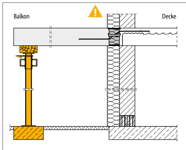
Abb. 163: Schöck Isokorb® XT Typ Q-ID: Stützung durchgängig erforderlich
