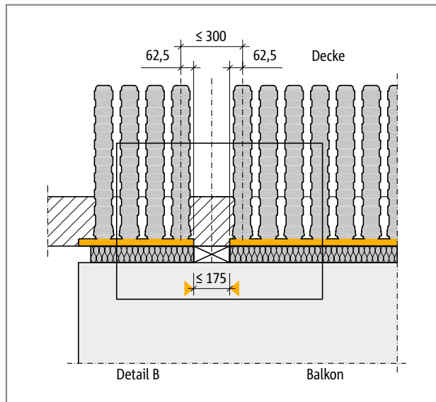
Abb. 115: Schöck Isokorb® T Typ K-ID: Anordnung einer Aussparung in der Dämmebene mit einer gewählten Länge \leq 175 mm
