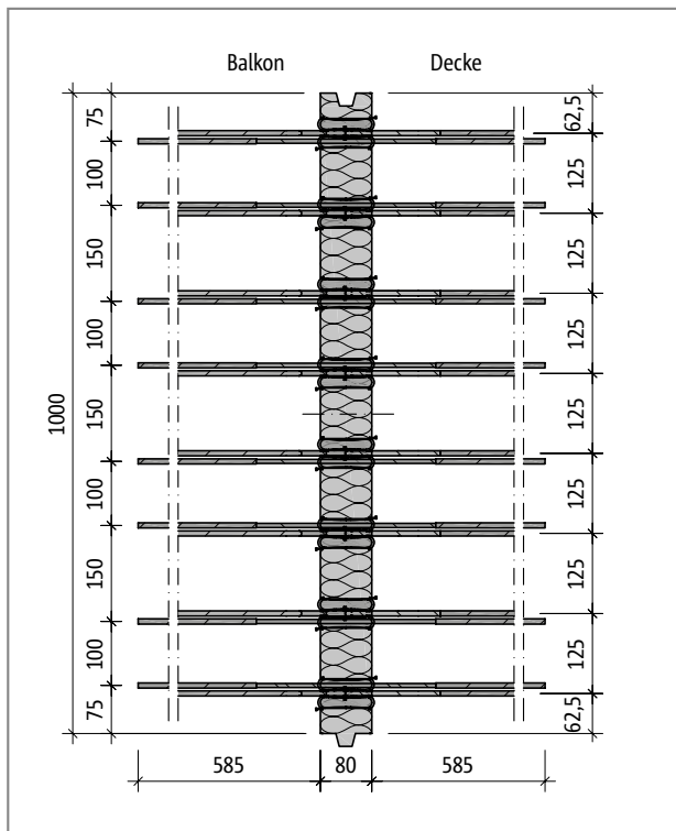
Abb. 119: Schöck Isokorb® T Typ K-ID-M1-V2-R0-X80: Produktgrundriss
