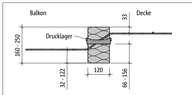
Abb. 156: Schöck Isokorb® XT Typ Q-ID-V1 bis V3 bei R0: Produktschnitt
