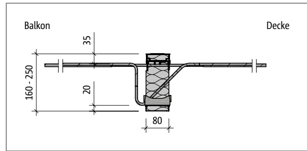
Abb. 126: Schöck Isokorb® T Typ K-ID-M2-V2-R0-X80: Produktschnitt
