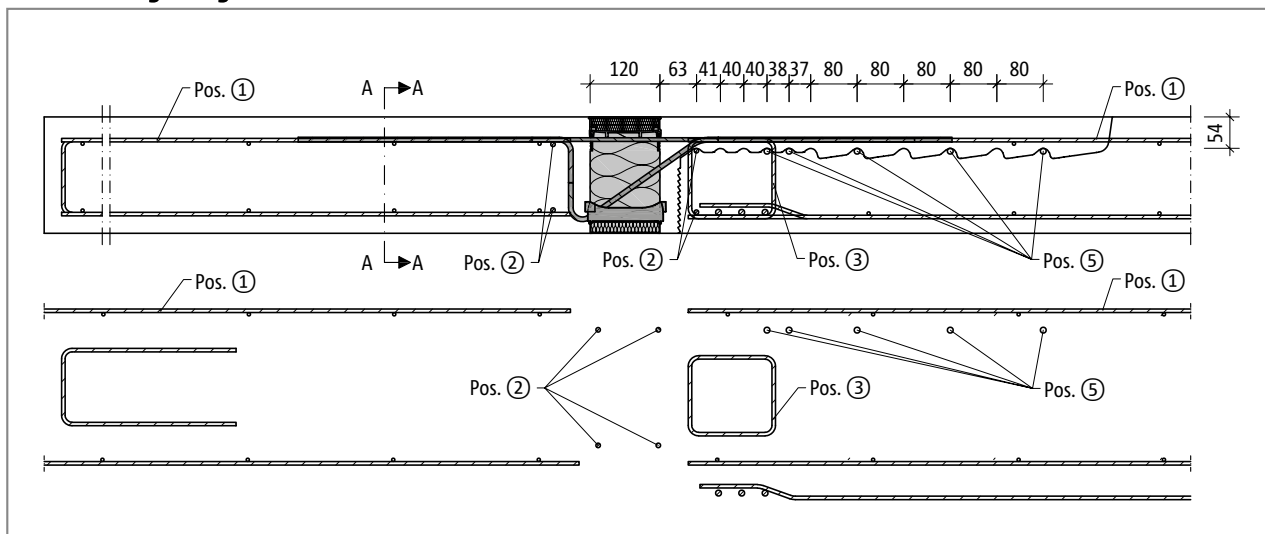
Abb. 90: Schöck Isokorb® XT Typ K-ID: Bauseitige Bewehrung bei indirekter Lagerung
