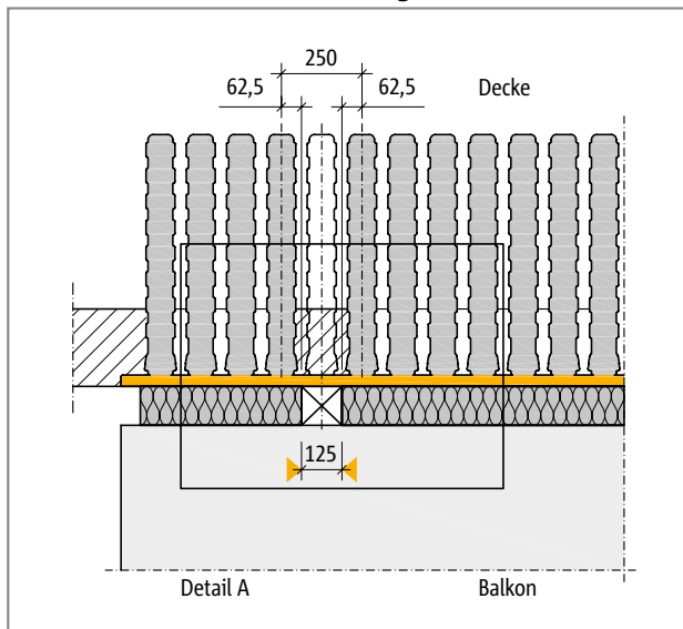
Abb. 148: Schöck Isokorb® XT Typ Q-ID: Anordnung einer Aussparung in der Dämmebene unter Berücksichtigung des Rastermaßes von 125 mm
