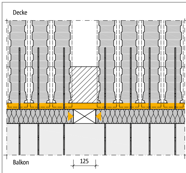
Abb. 177: Schöck Isokorb® T Typ Q-ID: Detail A, richtig durch Einhaltung des Rastermaßes und der vorgegebenen Abstände
