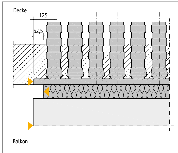
Abb. 174: Schöck Isokorb® T Typ Q-ID: Randabstand des Dämmkörpers, Achsmaß der Deckenaussparungen; Darstellung im Grundriss
