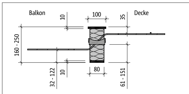
Abb. 180: Schöck Isokorb® T Typ Q-ID-V1-REI120-X80: Produktschnitt; der Produktschnitt entspricht auch den Haupttragstufen -V2, -V3
