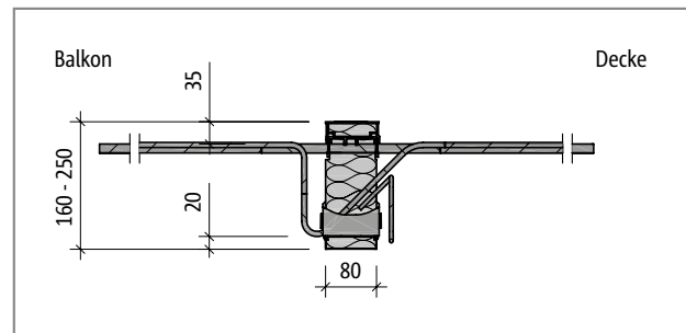
Abb. 128: Schöck Isokorb® T Typ K-ID-M4-V1-R0-X80: Produktschnitt
