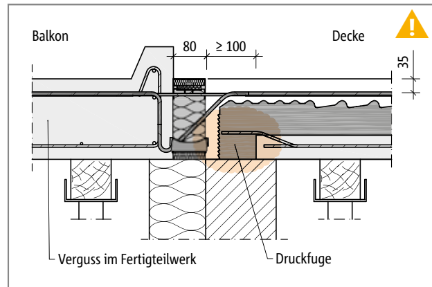
Abb. 135: Schöck Isokorb® T Typ K-ID: direkte Lagerung, Druckfuge deckenseitig
