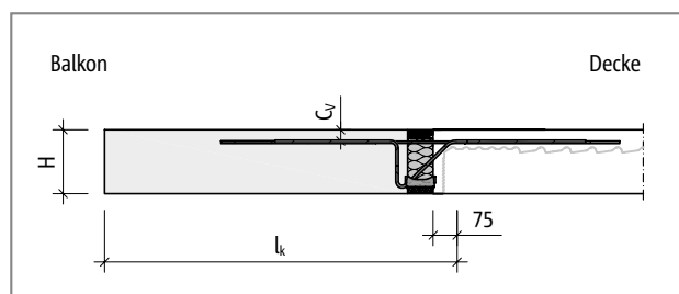
Abb. 108: Schöck Isokorb® T Typ K-ID: Bemessungswerte beziehen sich auf die dargestellte Kraglänge l_k bei direkter oder indirekter Lagerung
