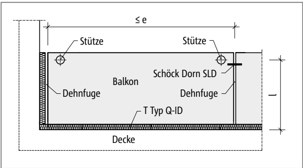
Abb. 173: Schöck Isokorb® T Typ Q-ID: Dehnfugenanordnung
