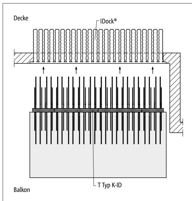
Abb. 14: Schöck Isokorb® Ausführungsvariante ID: Waagrechtes Einschieben des Balkons bei der Montage
