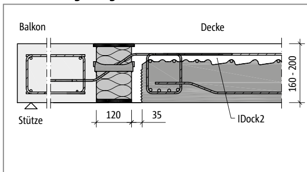
Abb. 143: Schöck Isokorb® XT Typ Q-ID: Anschluss von Balkonen mit Plattendicken von 160 mm bis 200 mm mit IDock2
