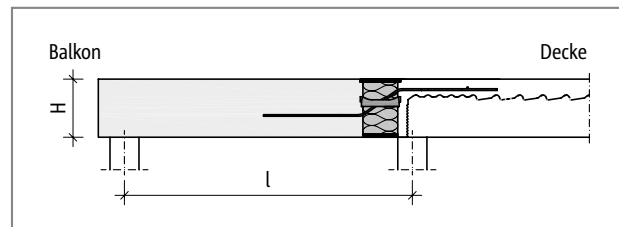
Abb. 144: Schöck Isokorb® XT Typ Q-ID: Statisches System
