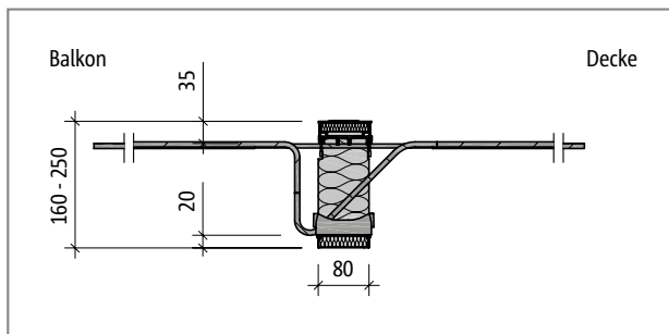
Abb. 117: Schöck Isokorb® T Typ K-ID-M1: Produktschnitt
