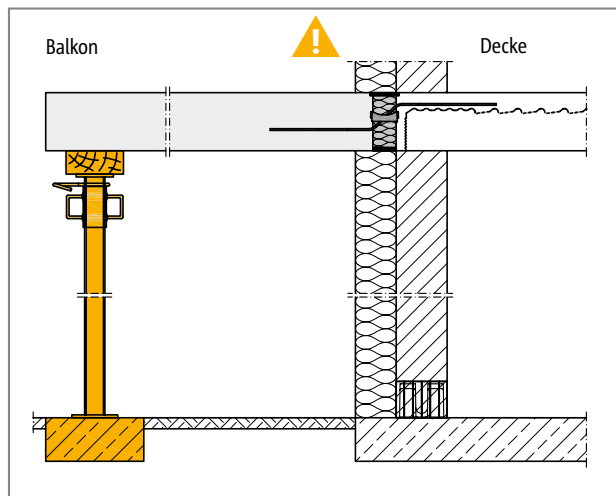
Abb. 191: Schöck Isokorb® T Typ Q-ID: Stützung durchgängig erforderlich
