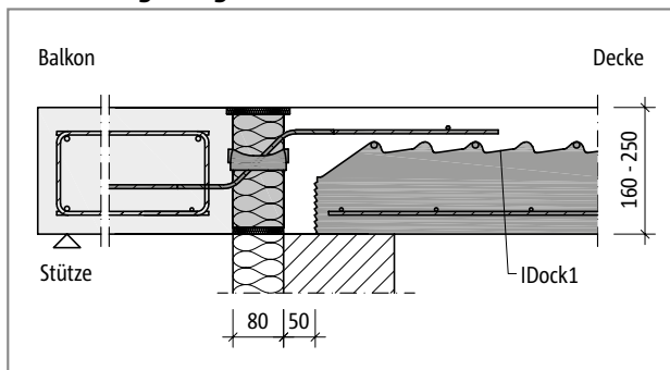
Abb. 170: Schöck Isokorb® T Typ Q-ID: Anschluss von Balkonen mit Plattendicken von 160 mm bis 250 mm mit IDock1
