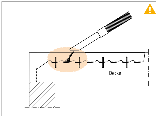
Abb. 194: Schöck IDock®: Gründliche Reinigung der Deckenaussparungen mit einem Staubsauger
