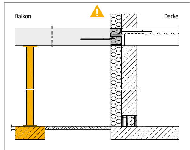
Abb. 164: Schöck Isokorb® XT Typ Q-ID: Stützung durchgängig erforderlich
