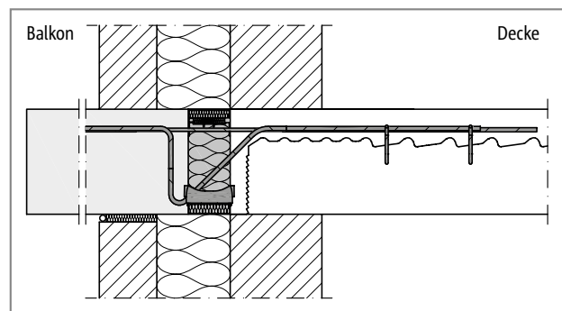
Abb. 102: Schöck Isokorb® T Typ K-ID: Anschluss bei Kerndämmung
