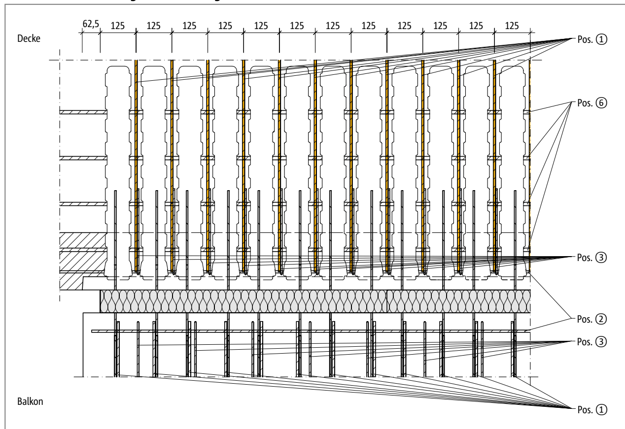
Abb. 186: Schöck Isokorb® T Typ Q-ID: Achsmaß der bauseitigen Bewehrung im Grundriss
