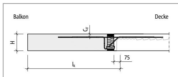
Abb. 107: Schöck Isokorb® T Typ K-ID: Bemessungswerte beziehen sich auf die dargestellte Kraglänge l_k bei direkter oder indirekter Lagerung
