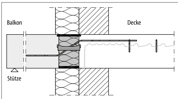
Abb. 138: Schöck Isokorb® XT Typ Q-ID: Anschluss bei Wärmedämmverbundsystem (WDVS)
