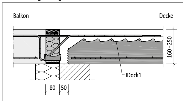
Abb. 105: Schöck Isokorb® T Typ K-ID: Anschluss von Balkonen mit Plattendicken von 160 mm bis 250 mm mit IDock1
