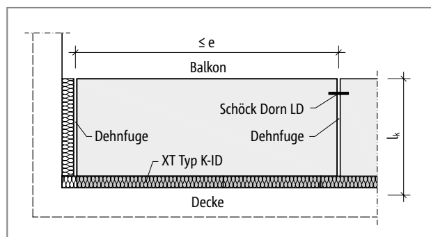
Abb. 67: Schöck Isokorb® XT Typ K-ID: Dehnfugenanordnung
