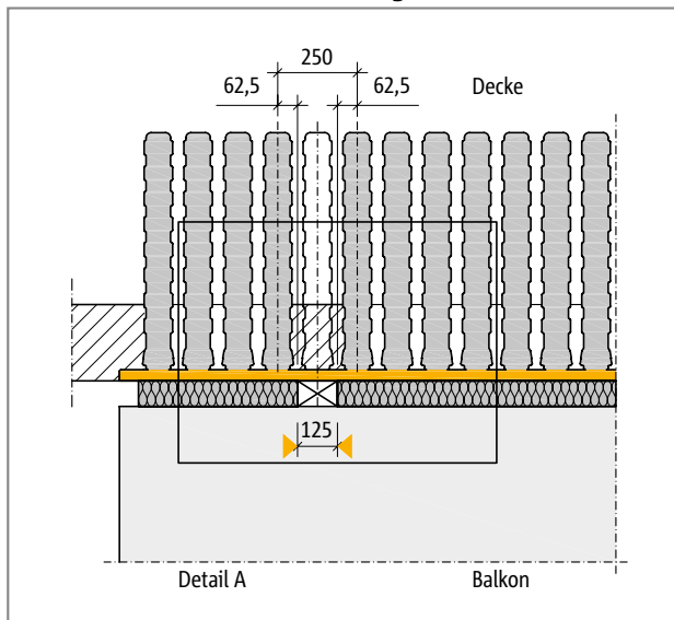
Abb. 113: Schöck Isokorb® T Typ K-ID: Anordnung einer Aussparung in der Dämmebene unter Berücksichtigung des Rastermaßes von 125 mm
