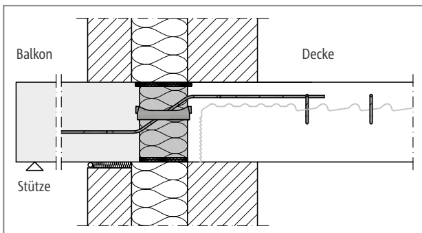
Abb. 140: Schöck Isokorb® XT Typ Q-ID: Anschluss bei zweischaligem Mauerwerk mit Kerndämmung
