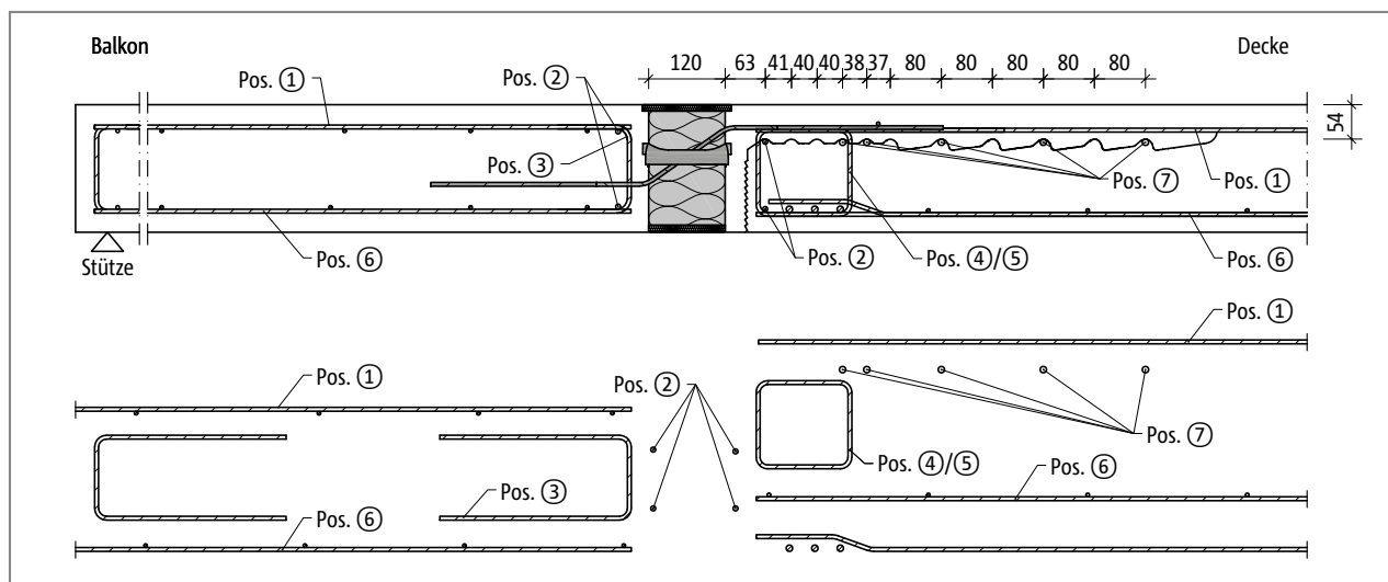
Abb. 162: Schöck Isokorb® XT Typ Q-ID: Bauseitige Bewehrung bei indirekter Lagerung; Beispiel Ortbetondecke
