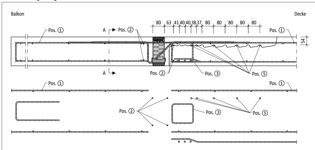
Abb. 133: Schöck Isokorb® T Typ K-ID: Bauseitige Bewehrung bei indirekter Lagerung
