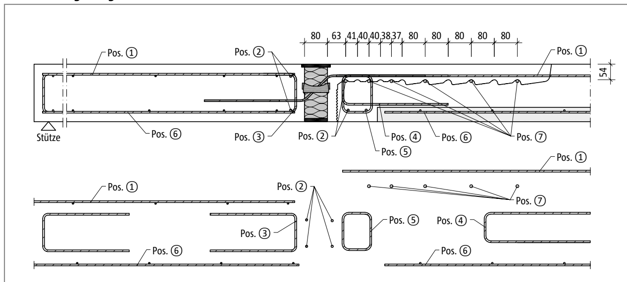
Abb. 189: Schöck Isokorb® T Typ Q-ID: Bauseitige Bewehrung bei indirekter Lagerung; Beispiel Elementdecke
