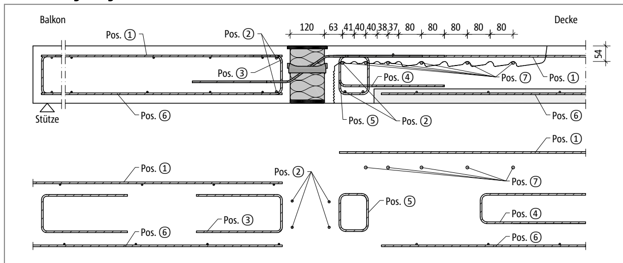
Abb. 161: Schöck Isokorb® XT Typ Q-ID: Bauseitige Bewehrung bei indirekter Lagerung; Beispiel Elementdecke
