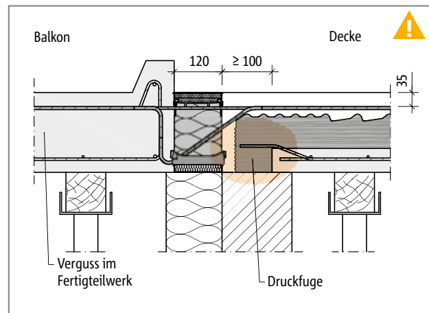
Abb. 92: Schöck Isokorb® XT Typ K-ID: direkte Lagerung, Druckfuge deckenseitig
