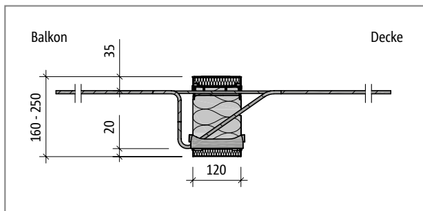
Abb. 74: Schöck Isokorb® XT Typ K-ID-M1: Produktschnitt
