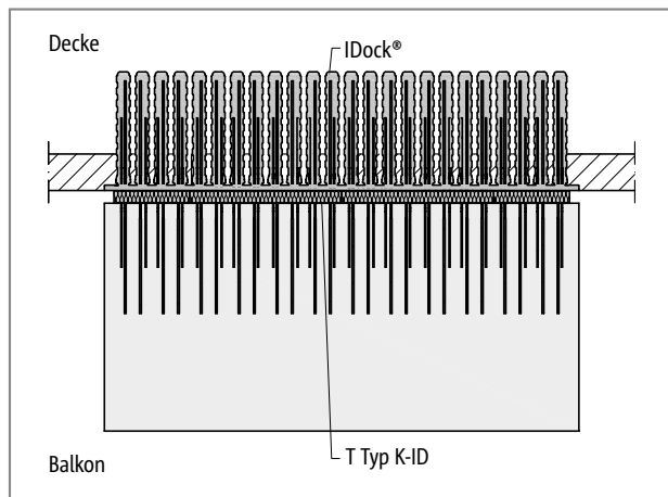
Abb. 96: Schöck Isokorb® T Typ K-ID: Balkon frei auskragend
