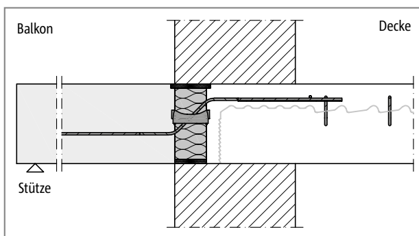
Abb. 167: Schöck Isokorb® T Typ Q-ID: Anschluss bei monolithischem Mauerwerk
