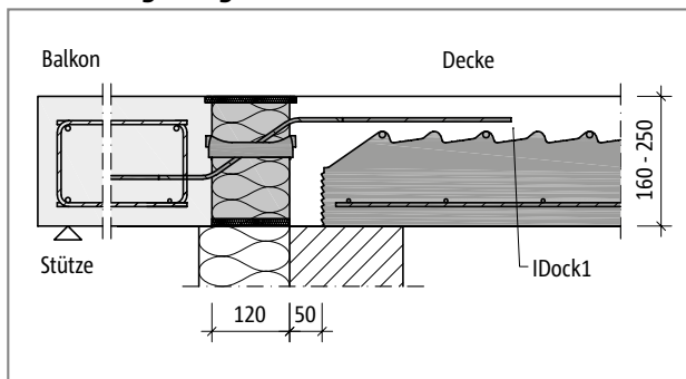
Abb. 142: Schöck Isokorb® XT Typ Q-ID: Anschluss von Balkonen mit Plattendicken von 160 mm bis 250 mm mit IDock1
