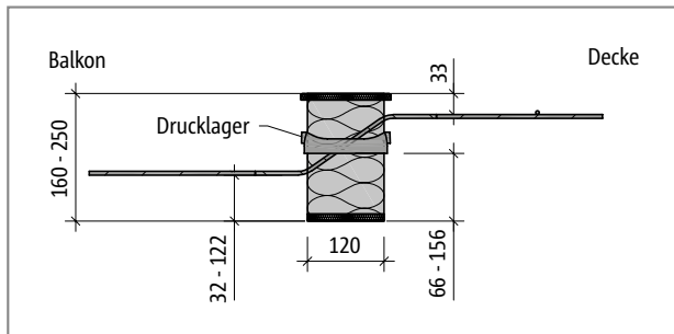
Abb. 152: Schöck Isokorb® XT Typ Q-ID-V1-REI120-X120: Produktschnitt; der Produktschnitt entspricht auch den Haupttragstufen -V2, -V3
