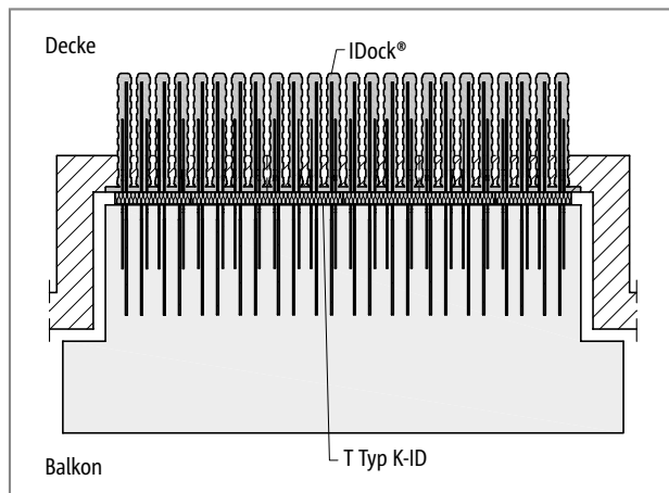
Abb. 98: Schöck Isokorb® T Typ K-ID: Balkon bei Fassadenrücksprung
