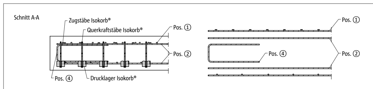
Abb. 130: Schöck Isokorb® T Typ K-ID: Bauseitige Bewehrung balkonseitig im Schnitt A-A; Pos. 4 = konstruktive Randeinfassung am freien Rand
