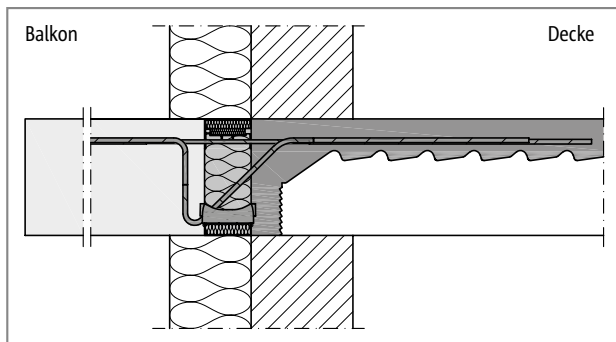
Abb. 103: Schöck Isokorb® T Typ K-ID: Anschluss mit IDock1 bis zur Isokorb® Höhe H250 möglich; Dämmung durch WDVS
