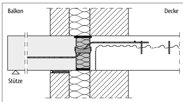
Abb. 168: Schöck Isokorb® T Typ Q-ID: Anschluss bei Kerndämmung
