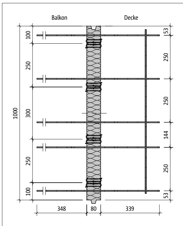
Abb. 182: Schöck Isokorb® T Typ Q-ID-V1-REI120-X80: Produktgrundriss
