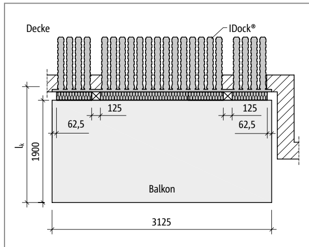
Abb. 93: Schöck Isokorb® XT Typ K-ID: Grundriss
