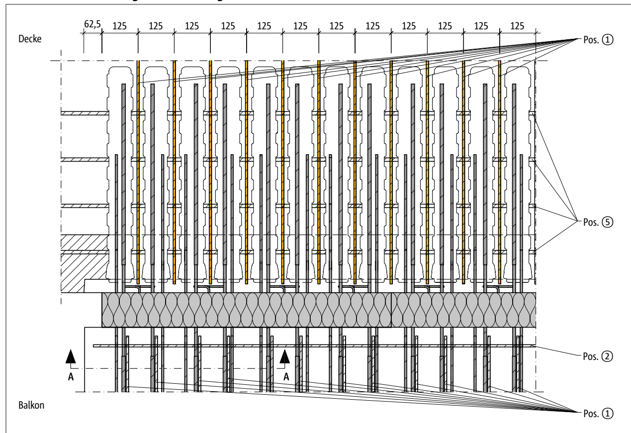
Abb. 86: Schöck Isokorb® XT Typ K-ID: Achsmaß der bauseitigen Bewehrung im Grundriss
