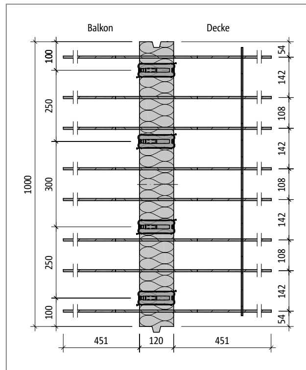
Abb. 155: Schöck Isokorb® XT Typ Q-ID-V4: Produktgrundriss
