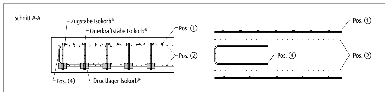
Abb. 87: Schöck Isokorb® XT Typ K-ID: Bauseitige Bewehrung balkonseitig im Schnitt A-A; Pos. 4 = konstruktive Randeinfassung am freien Rand
