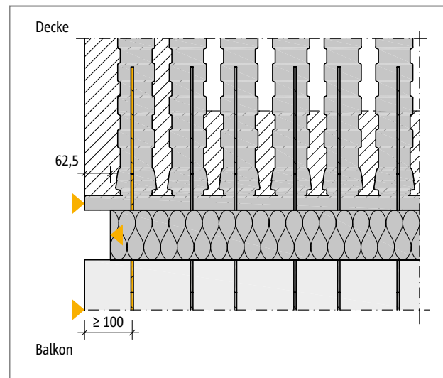
Abb. 147: Schöck Isokorb® XT Typ Q-ID: Randabstand des Dämmkörpers, Mindestabstand des Querkraftstabs; Darstellung im Grundriss
