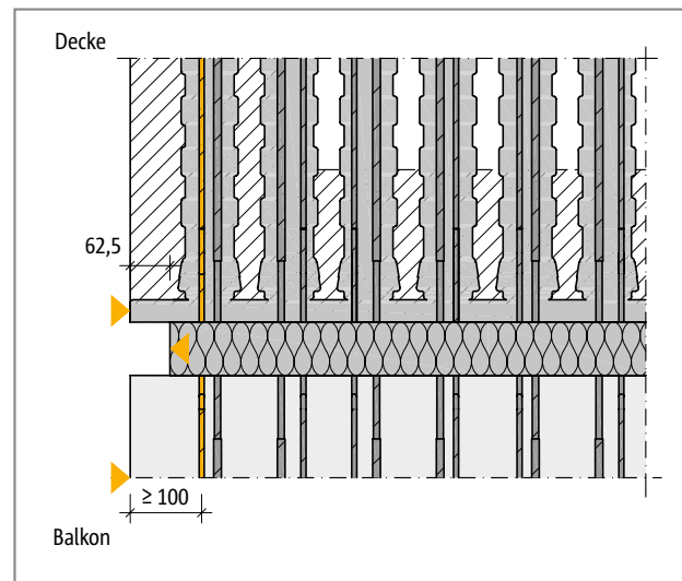
Abb. 112: Schöck Isokorb® T Typ K-ID: Randabstand des Dämmkörpers, Mindestrandabstand des Querkraftstabs; Darstellung im Grundriss
