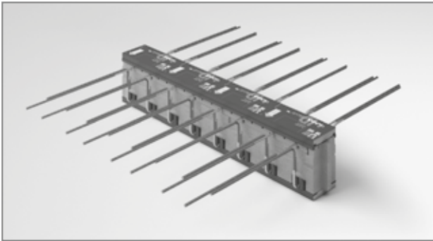
Abb. 1: Schöck Isokorb® Ausführungsvante ID
