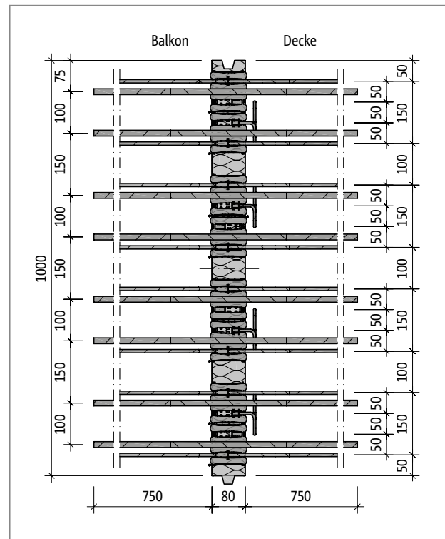
Abb. 124: Schöck Isokorb® T Typ K-ID-M4-V1-R0-X80: Produktgrundriss
