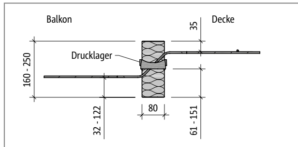
Abb. 184: Schöck Isokorb® T Typ Q-ID-V1-R0-X80: Produktschnitt; der Produktschnitt entspricht auch den Haupttragstufen -V2, -V3
