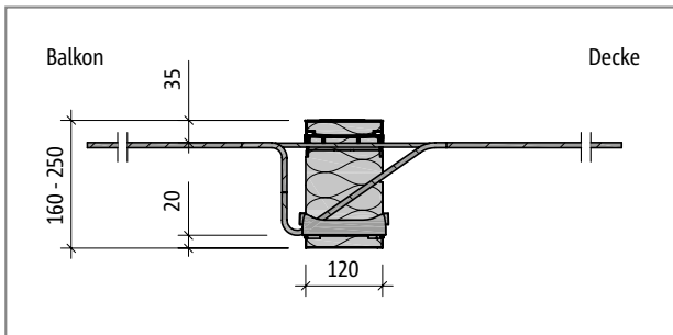
Abb. 82: Schöck Isokorb® XT Typ K-ID-M1 bei R0: Produktschnitt
