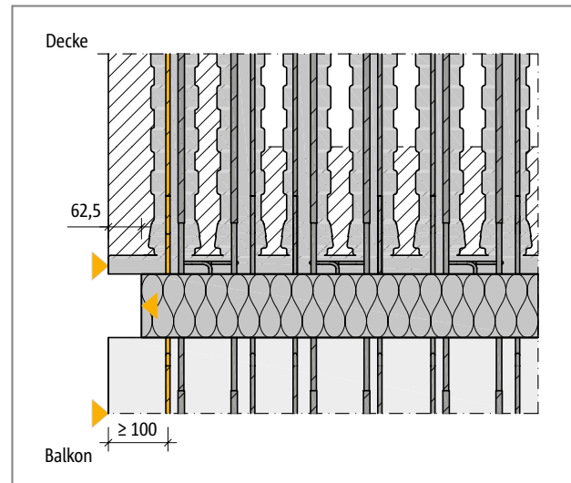
Abb. 69: Schöck Isokorb® XT Typ K-ID: Randabstand des Dämmkörpers, Mindestrandabstand des Querkraftstabs; Darstellung im Grundriss
