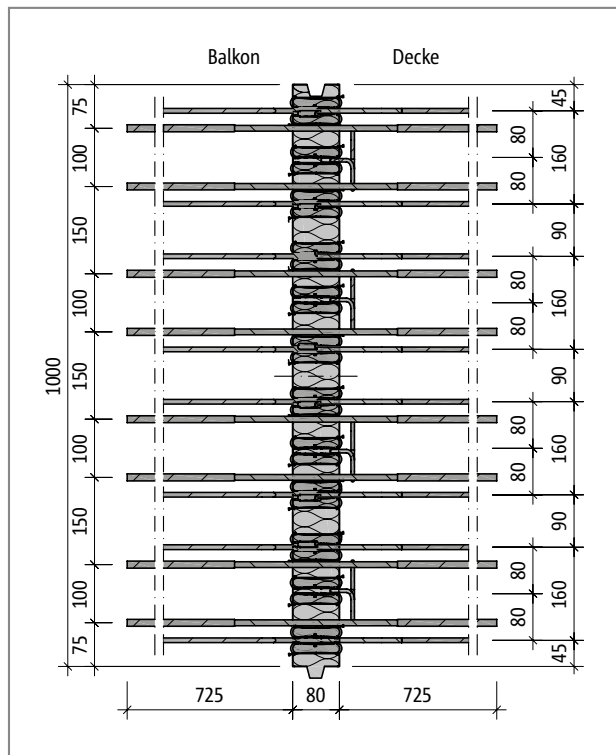
Abb. 123: Schöck Isokorb® T Typ K-ID-M3-V2-R0-X80: Produktgrundriss
