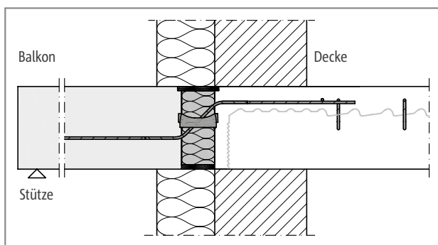
Abb. 166: Schöck Isokorb® T Typ Q-ID: Anschluss bei Außendämmung
