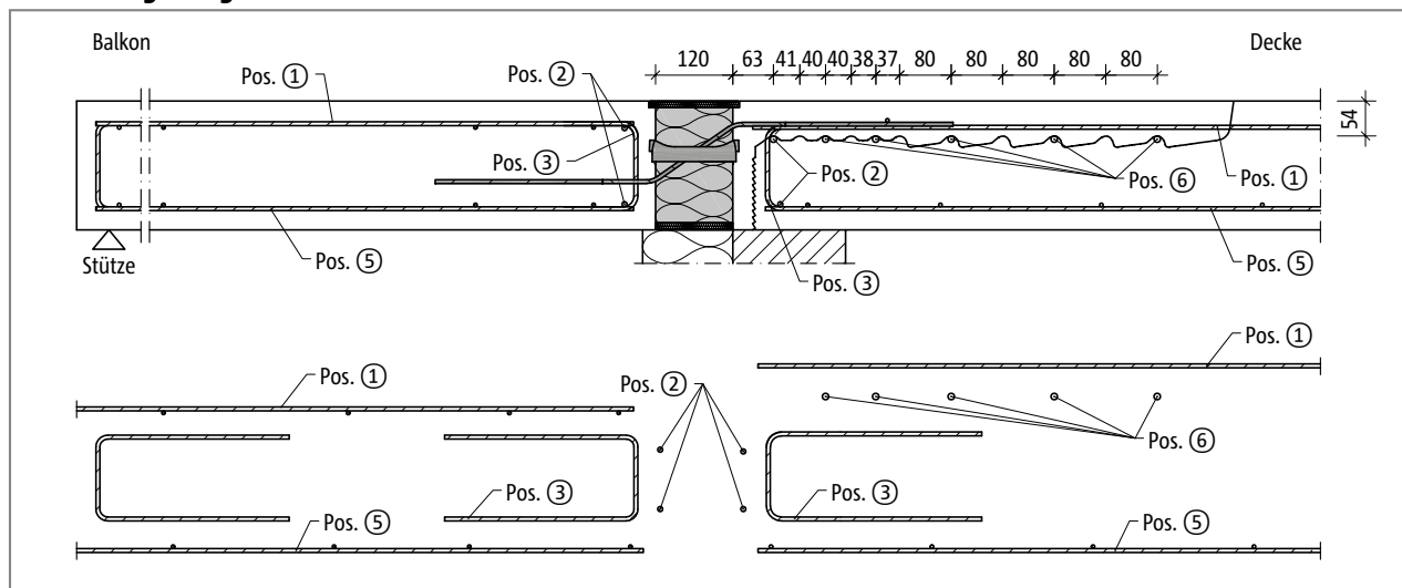
Abb. 160: Schöck Isokorb® XT Typ Q-ID: Bauseitige Bewehrung bei direkter Lagerung
