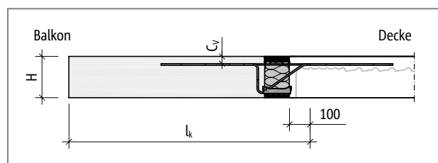
Abb. 64: Schöck Isokorb® XT Typ K-ID: Bemessungswerte beziehen sich auf die dargestellte Kraglänge l_k bei direkter oder indirekter Lagerung
