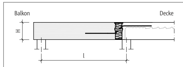
Abb. 172: Schöck Isokorb® T Typ Q-ID: Statisches System
