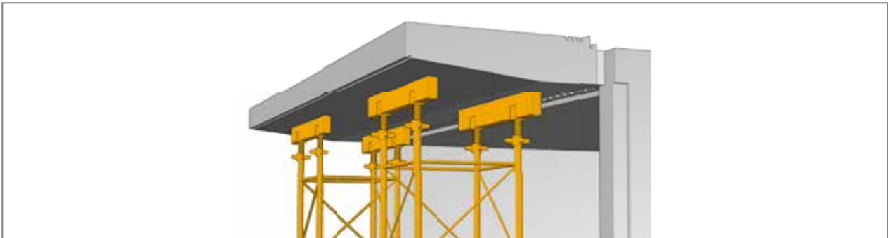
Abb. 195: Schöck IDock®: Abstützung des Vollfertigteilbalkons auf dem darunterliegenden Balkon
