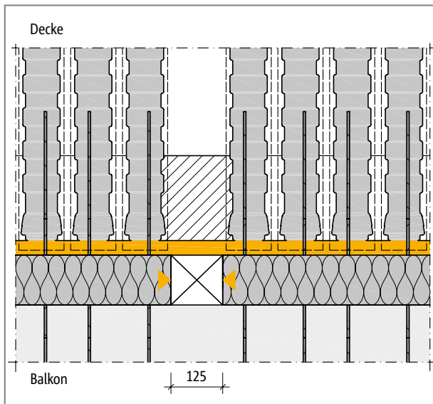
Abb. 149: Schöck Isokorb® XT Typ Q-ID: Detail A, richtig durch Einhaltung des Rastermaßes und der vorgegebenen Abstände
