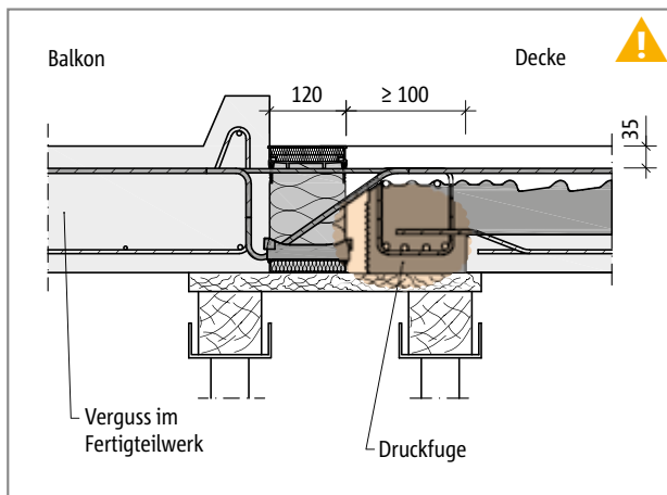
Abb. 91: Schöck Isokorb® XT Typ K-ID: indirekte Lagerung, Druckfuge deckenseitig
