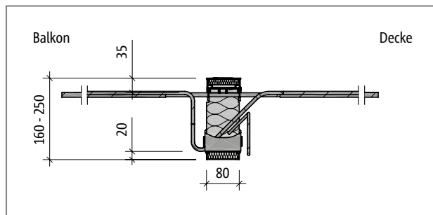
Abb. 121: Schöck Isokorb® T Typ K-ID-M3: Produktschnitt
