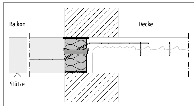
Abb. 139: Schöck Isokorb® XT Typ Q-ID: Anschluss bei einschaligem, wärmedämmendem Mauerwerk
