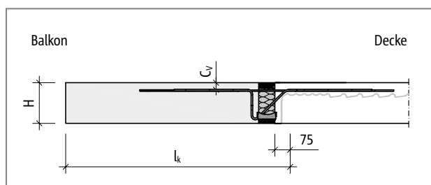
Abb. 109: Schöck Isokorb® T Typ K-ID: Bemessungswerte beziehen sich auf die dargestellte Kraglänge l_k bei direkter oder indirekter Lagerung
