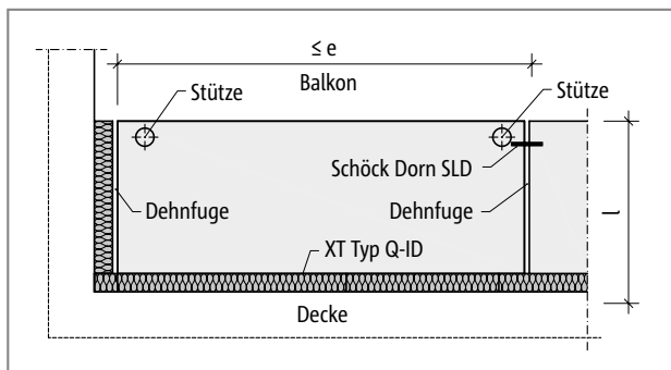
Abb. 145: Schöck Isokorb® XT Typ Q-ID: Dehnfugenanordnung
