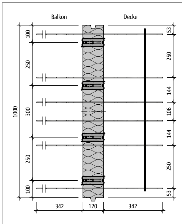
Abb. 154: Schöck Isokorb® XT Typ Q-ID-V2: Produktgrundriss
