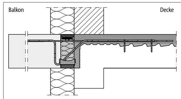
Abb. 104: Schöck Isokorb® T Typ K-ID: Anschluss mit IDock2 bis zur Isokorb® Höhe H200 möglich; Darstellung mit Randunterzug und WDVS
