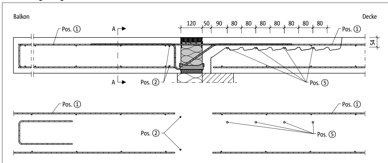
Abb. 88: Schöck Isokorb® XT Typ K-ID: Bauseitige Bewehrung bei direkter Lagerung
