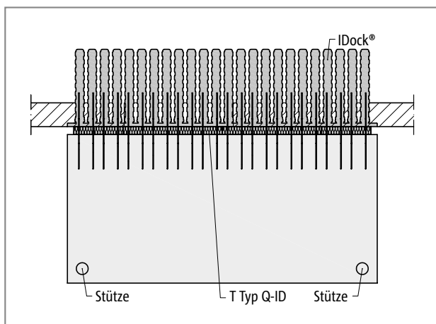
Abb. 165: Schöck Isokorb® T Typ Q-ID: Balkon mit Stützenlagerung
