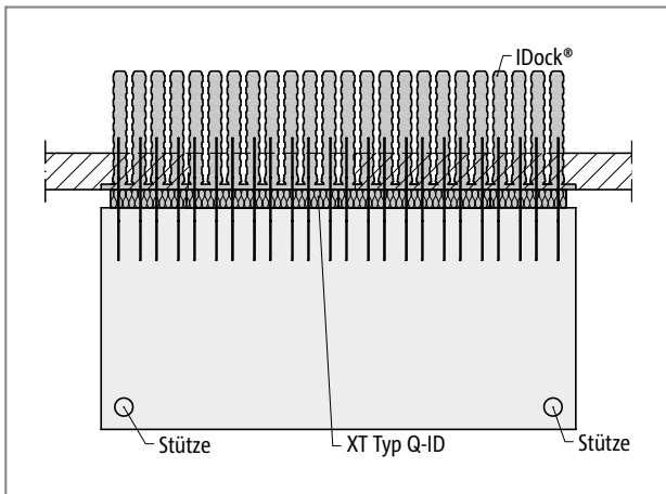
Abb. 137: Schöck Isokorb® XT Typ Q-ID: Balkon mit Stützenlagerung
