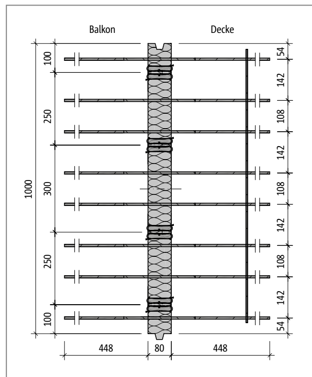
Abb. 183: Schöck Isokorb® T Typ Q-ID-V4-REI120-X80: Produktgrundriss
