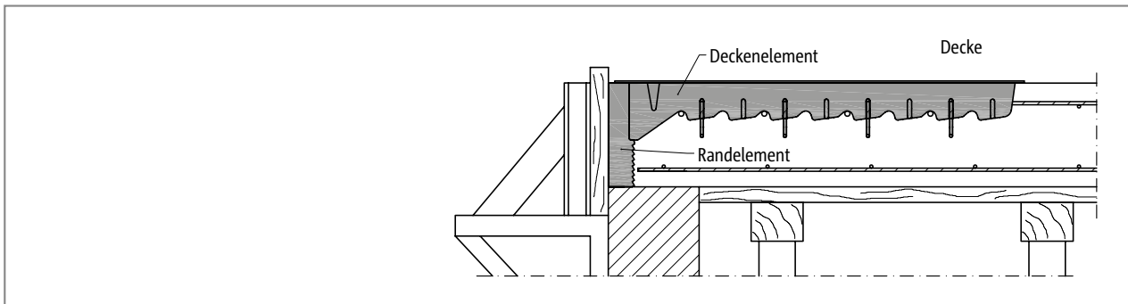
Abb. 24: Schöck IDock®: IDock1, Außenwand als direktes Auflager; die Deckenaussparung wird durch die beiden Komponenten Randelement und Deckenelement abgesichert
