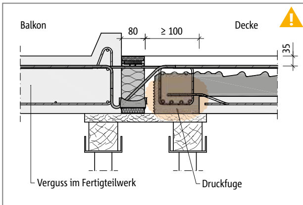
Abb. 134: Schöck Isokorb® T Typ K-ID: indirekte Lagerung, Druckfuge deckenseitig
