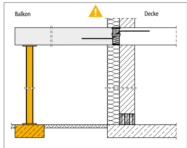
Abb. 192: Schöck Isokorb® T Typ Q-ID: Stützung durchgängig erforderlich
