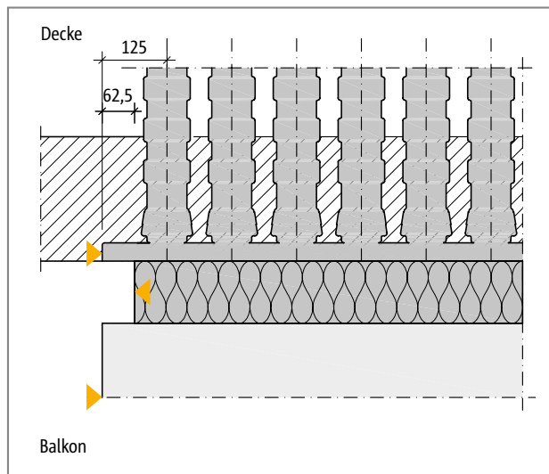
Abb. 146: Schöck Isokorb® XT Typ Q-ID: Randabstand des Dämmkörpers, Achsmaß der Deckenaussparungen; Darstellung im Grundriss
