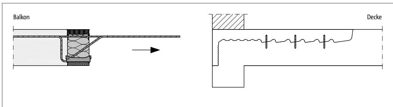
Abb. 28: Schöck IDock®: Waagrechtes Einschieben des Fertigteil-Balkons mit dem einbetonierten Schöck Isokorb® Ausführungsvariante ID; die Zug- und Querkraftstäbe des Isokorb® finden in den Deckenaussparungen Platz
