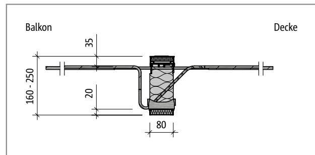
Abb. 118: Schöck Isokorb® T Typ K-ID-M2: Produktschnitt
