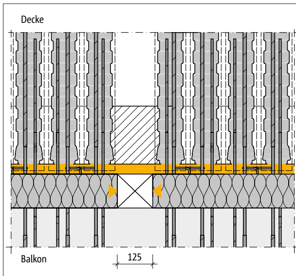
Abb. 71: Schöck Isokorb® XT Typ K-ID: Detail A, richtig durch Einhaltung des Rastermaßes und der vorgegebenen Abstände
