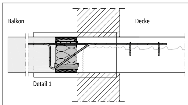
Abb. 3: Schöck Isokorb® XT Typ K-ID bei REI120: Brandschutzplatte oben und unten; seitlich integrierte Brandschutzbänder
