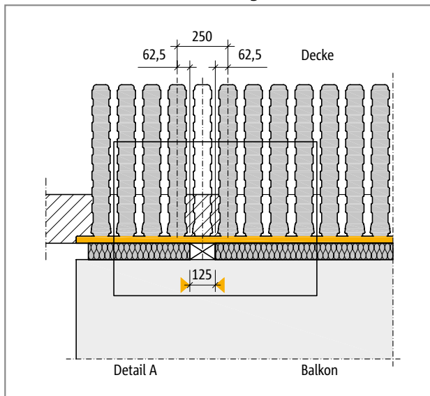
Abb. 176: Schöck Isokorb® T Typ Q-ID: Anordnung einer Aussparung in der Dämmebene unter Berücksichtigung des Rastermaßes von 125 mm
