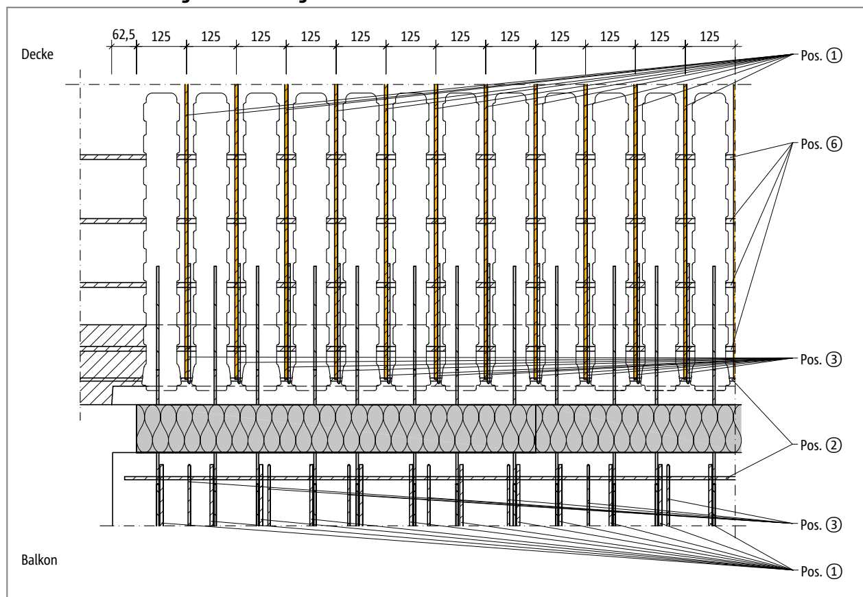
Abb. 158: Schöck Isokorb® XT Typ Q-ID: Achsmaß der bauseitigen Bewehrung im Grundriss
