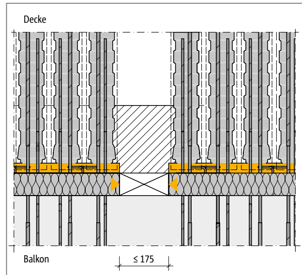
Abb. 116: Schöck Isokorb® T Typ K-ID: Detail B, richtig durch Einhaltung der vorgegebenen Abstände und der Aussparungslänge \leq 175 mm
