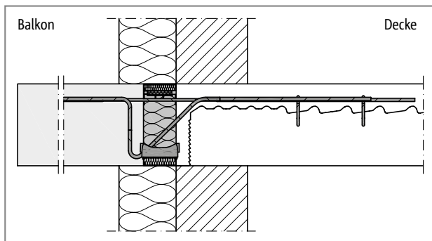
Abb. 99: Schöck Isokorb® T Typ K-ID: Anschluss bei Wärmedämmverbundsystem (WDVS)
