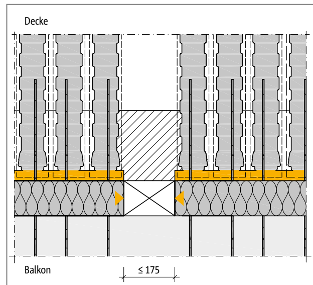
Abb. 151: Schöck Isokorb® XT Typ Q-ID: Detail B, richtig durch Einhaltung der vorgegebenen Abstände und der Aussparungslänge \leq 175 mm
