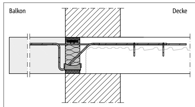
Abb. 100: Schöck Isokorb® T Typ K-ID: Anschluss bei monolithischem Mauerwerk
