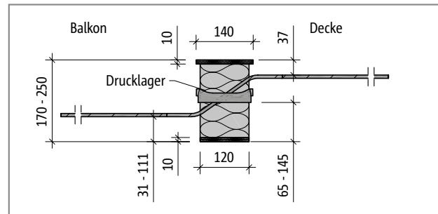
Abb. 153: Schöck Isokorb® XT Typ Q-ID-V4-REI120-X120: Produktschnitt
