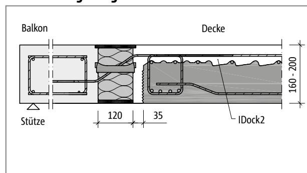
Abb. 31: Schöck IDock®: Anschluss von Balkonen mit Plattendicken von 160 mm bis 200 mm mit IDock2
