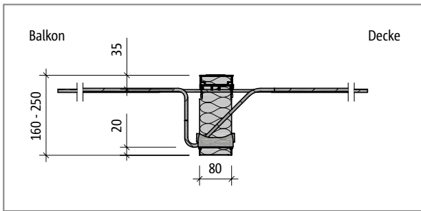
Abb. 125: Schöck Isokorb® T Typ K-ID-M1-V2-R0-X80: Produktschnitt
