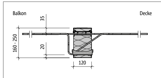
Abb. 83: Schöck Isokorb® XT Typ K-ID-M2 bei R0: Produktschnitt
