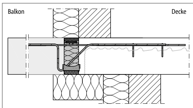
Abb. 101: Schöck Isokorb® T Typ K-ID: Anschluss bei indirekt gelagerter Decke und WDVS
