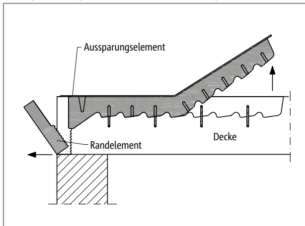
Abb. 193: Schöck IDock®: Entfernung der Rand- und Aussparungselemente vor der Balkon-Montage
