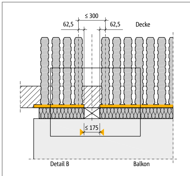
Abb. 72: Schöck Isokorb® XT Typ K-ID: Anordnung einer Aussparung in der Dämmebene mit einer gewählten Länge \leq 175 mm
