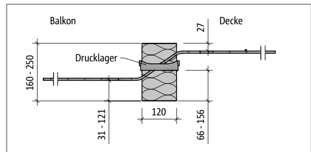
Abb. 157: Schöck Isokorb® XT Typ Q-ID-V4 bei R0: Produktschnitt
