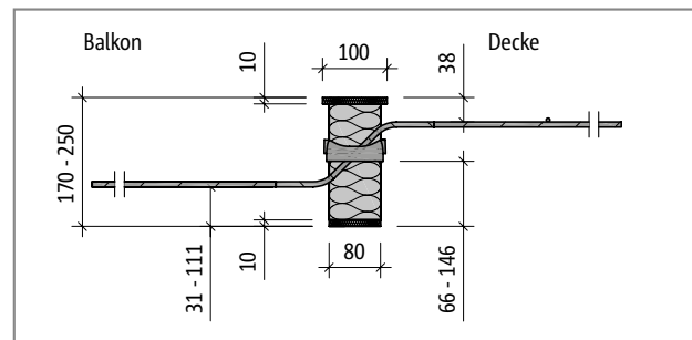
Abb. 181: Schöck Isokorb® T Typ Q-ID-V4-REI120-X80: Produktschnitt
