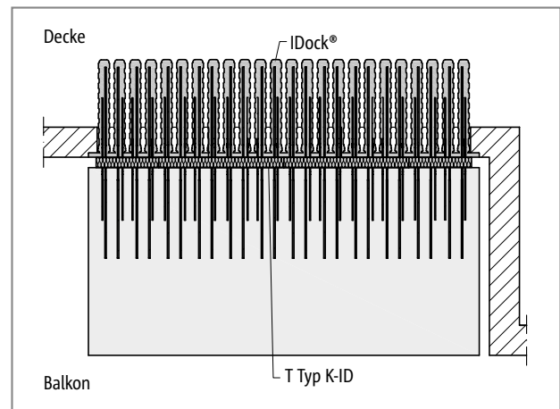
Abb. 97: Schöck Isokorb® T Typ K-ID: Balkon bei Fassadenversprung
