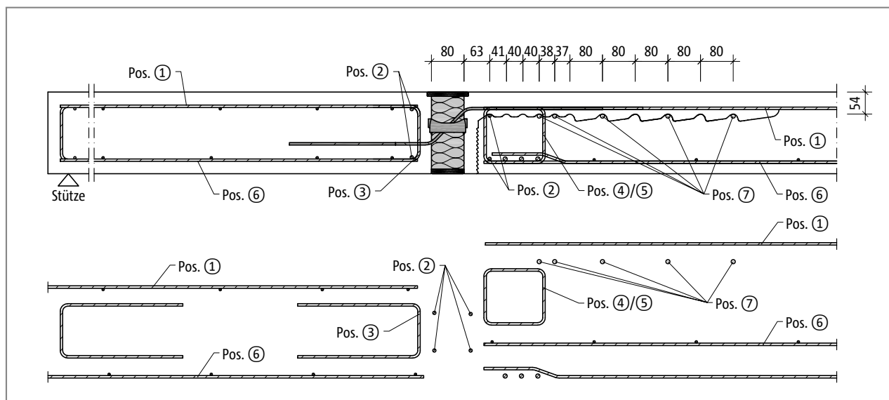
Abb. 190: Schöck Isokorb® T Typ Q-ID: Bauseitige Bewehrung bei indirekter Lagerung; Beispiel Ortbetondecke
