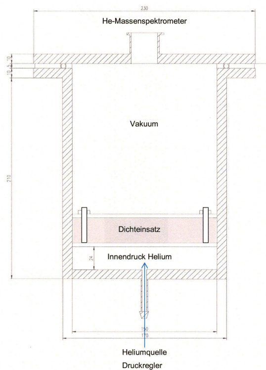
Bild 2: Prüfeinrichtung (schematisch)
