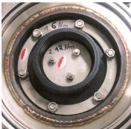
Bild 1: Dichteinsatz im Einbauszustand
