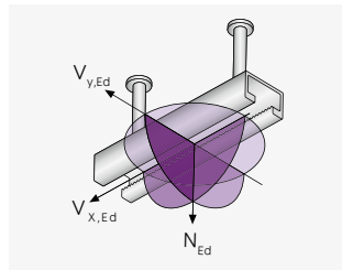
Bild a) JXA, JXA Einzellasten (für alle Lastrichtungen)
